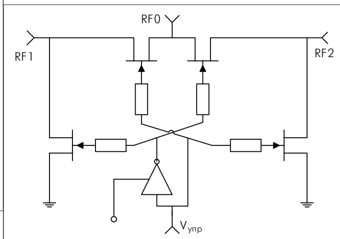
Рис.9. Принципиальная электрическая схема КМОП-переключателя на полевых транзисторах фирмы Peregrine Semiconductor
