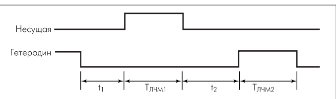
Рис. 1. Временные диаграммы работы синтезатора
