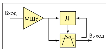
Рис.4. Структурная схема фильтра с автоподстройкой на несущую частоту входного сигнала
