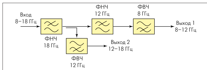
Рис.3. Структура диплексора на полосу частот 8–18 ГГц
