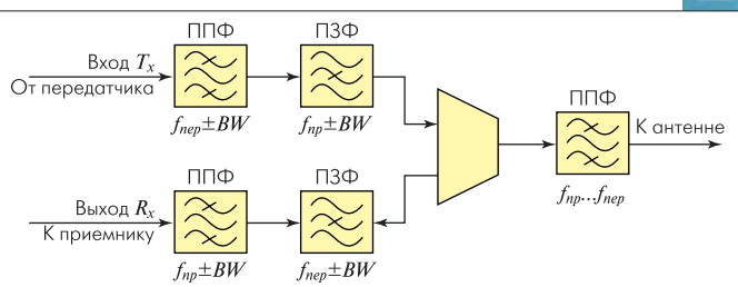
Рис.5. Структурная схема дуплексера
