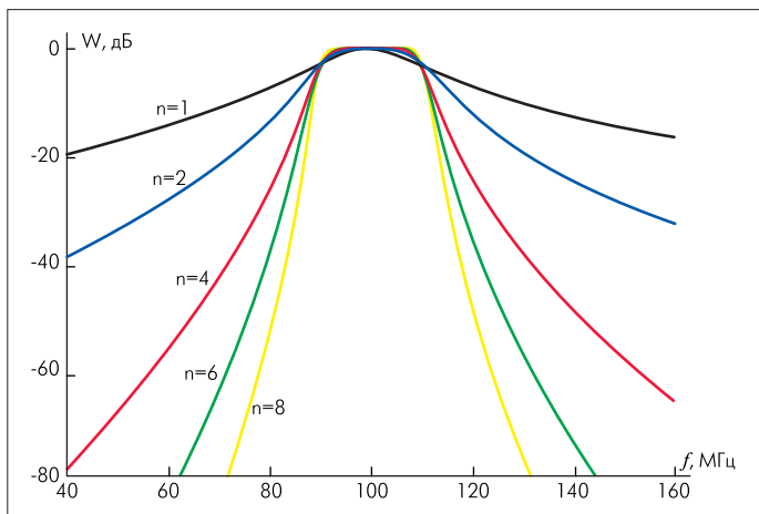
Рис.2. Амплитудно-частотные характеристики ППФ Баттерворта на полосу частот 90–110 МГц с различным числом звеньев
