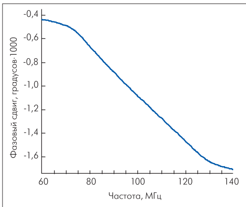
Рис.1. Фазочастотная характеристика восьмизвонного ППФ, настроенного на ее высокую линейность
