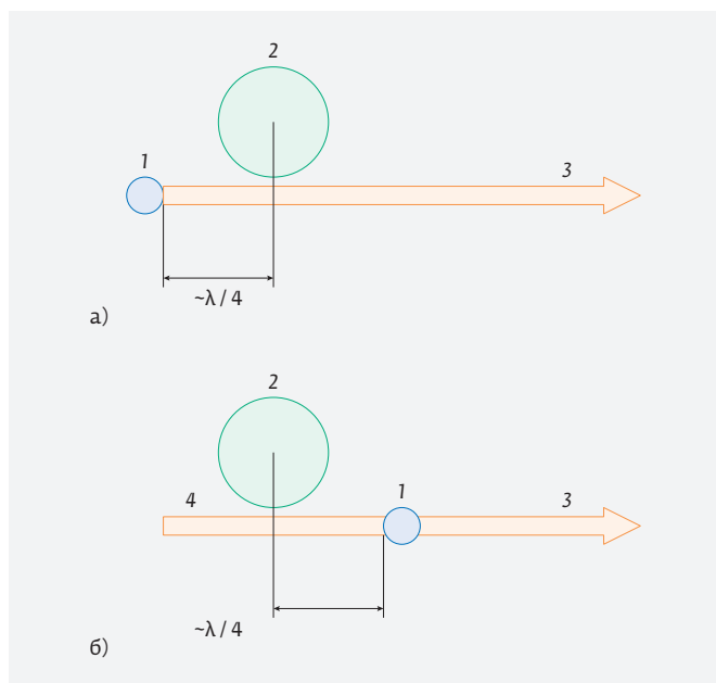
Рис. 6. Схематическое изображение топологий микрополосковых диодных автогенераторов с ДР 2: а – ДР в линии 3 вывода мощности, б – диодный генератор с реактивно отражающим резонатором 4
