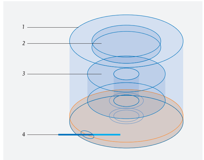
Рис. 2. Условный вид колебательной системы с ДР с цилиндрическим экраном, возбуждаемой коаксиальной линией: 1 – экранируемая полость; 2 – диск перестройки частоты ДР; 3 – ДР; 4 – элемент возбуждения колебаний ДР
