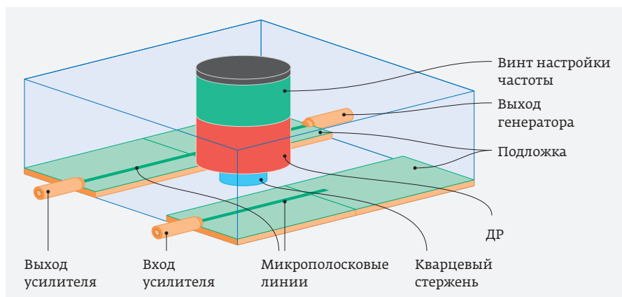
Рис. 13. Вид модели колебательной системы
