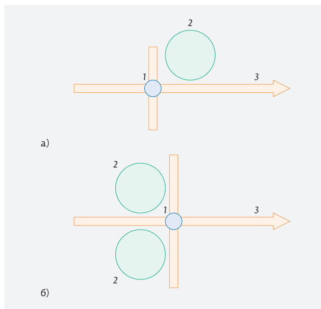
Рис. 7. Схематическое изображение топологий микрополосковых транзисторных автогенераторов с колебательной системой на ДР 2: а – ДР в линии 3 вывода мощности, б – ППФ между базой и эмиттером
