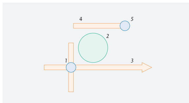
Рис. 19. Схематическое изображение топологии микрополоскового транзисторного автогенератора с колебательной системой на ДР, перестраиваемого варакторным диодом: 1 – транзистор; 2 – ДР; 3 – линия вывода мощности; 4 – отрезок микрополосковой линии для управления частотой колебательной системы; 5 – варакторный диод
