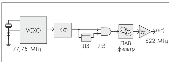
Рис.4. Схема умножения частоты колебаний базового управляемого напряжением кварцевого генератора модели VC-700&VS-720
