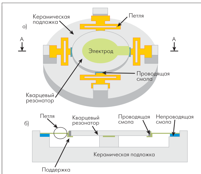
Рис.1. Вид сверху (а) и в сечении AA (б) кварцевого резонатора типа HFF
