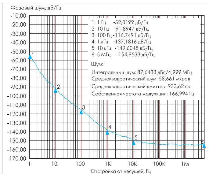
Рис.5. Характеристика СПМ фазового шума VCS4 вблизи частоты 2,5 МГц
