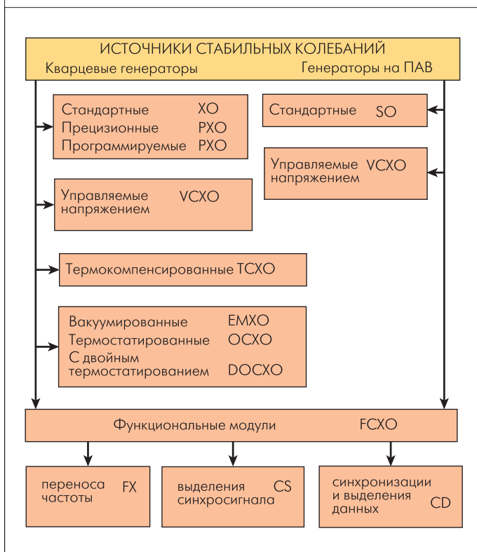
Рис.2. Классификация кварцевых и ПАВ-генераторов компании Vectron International
