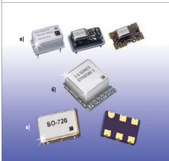
Рис.3. Генераторы классов XO (а), PXO (б) и SO (в)
