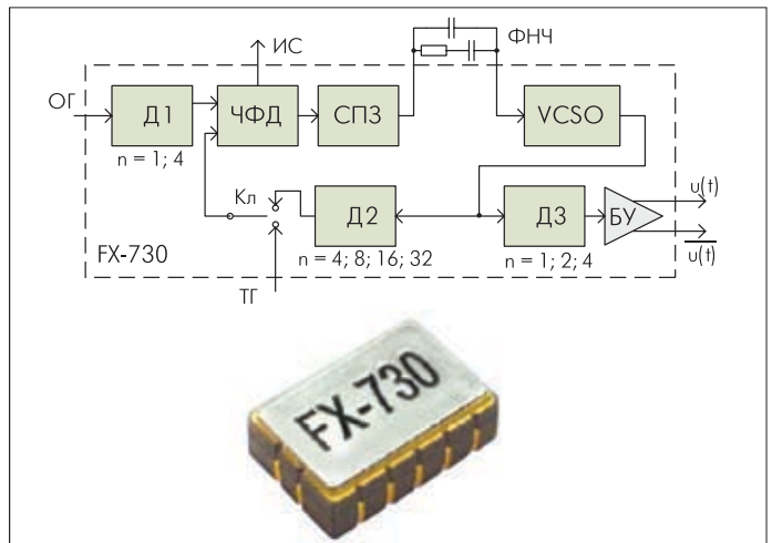
Рис.6. Структурная схема (а) и внешний вид (б) преобразователя частот FX-730: Д1, Д2, Д3 – делители частоты, ЧФД – частотно-фазовый детектор, СПЗ – схема подкачки заряда (Charge Pump), ФНЧ – внешние элементы фильтра нижних частот; БУ – буферный усилитель; КЛ – ключ, ИС – выход на индикатор синхронизма; ОГ – генератор опорного сигнала; ТГ – генератор тактового сигнала
