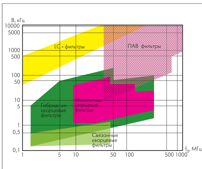
Рис.7. Средняя частота и полоса пропускания частотных фильтров, выполненных по различной технологии
