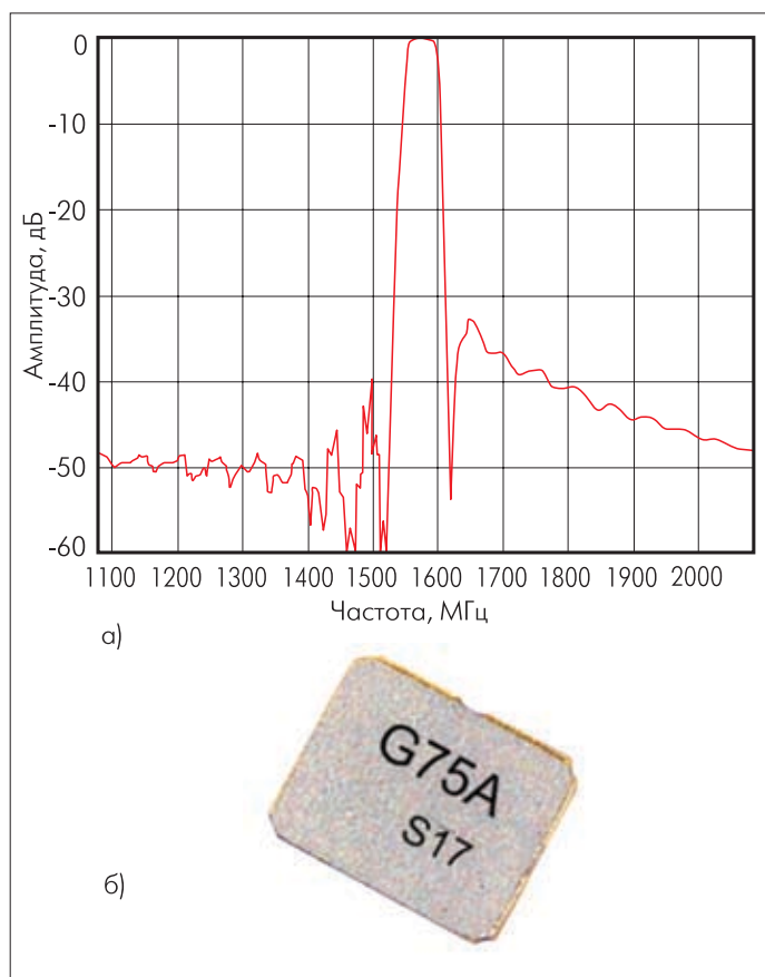
Рис. 8. АЧХ (а) и внешний вид (б) ПАВ-фильтра (средняя частота 1575 МГц, полоса 2 МГц, потери в полосе прозрачности 1,5 дБ, габариты 2,5×2 мм)
