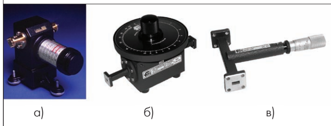
Рис.7. Волноводные модели измерительных аттенюаторов компаний Millitech (а) и Flann Microwave серий 114 (б) и 020 (в)
