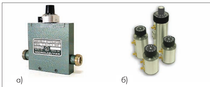
Рис.6. Измерительные коаксиальные аттенюаторы с ручным управлением: AJ-41 компании Microlab/FXR (а) и BMA35111 с роторной установкой ослабления компании Trilithic (б)
