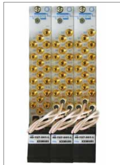
▲ Рис. 6. Матрица в конфигурации 48×4, полученная с помощью соединения трех матриц с конфигурацией 16×4 (модель 40-727-001-L) для рабочих частот до 300 МГц
